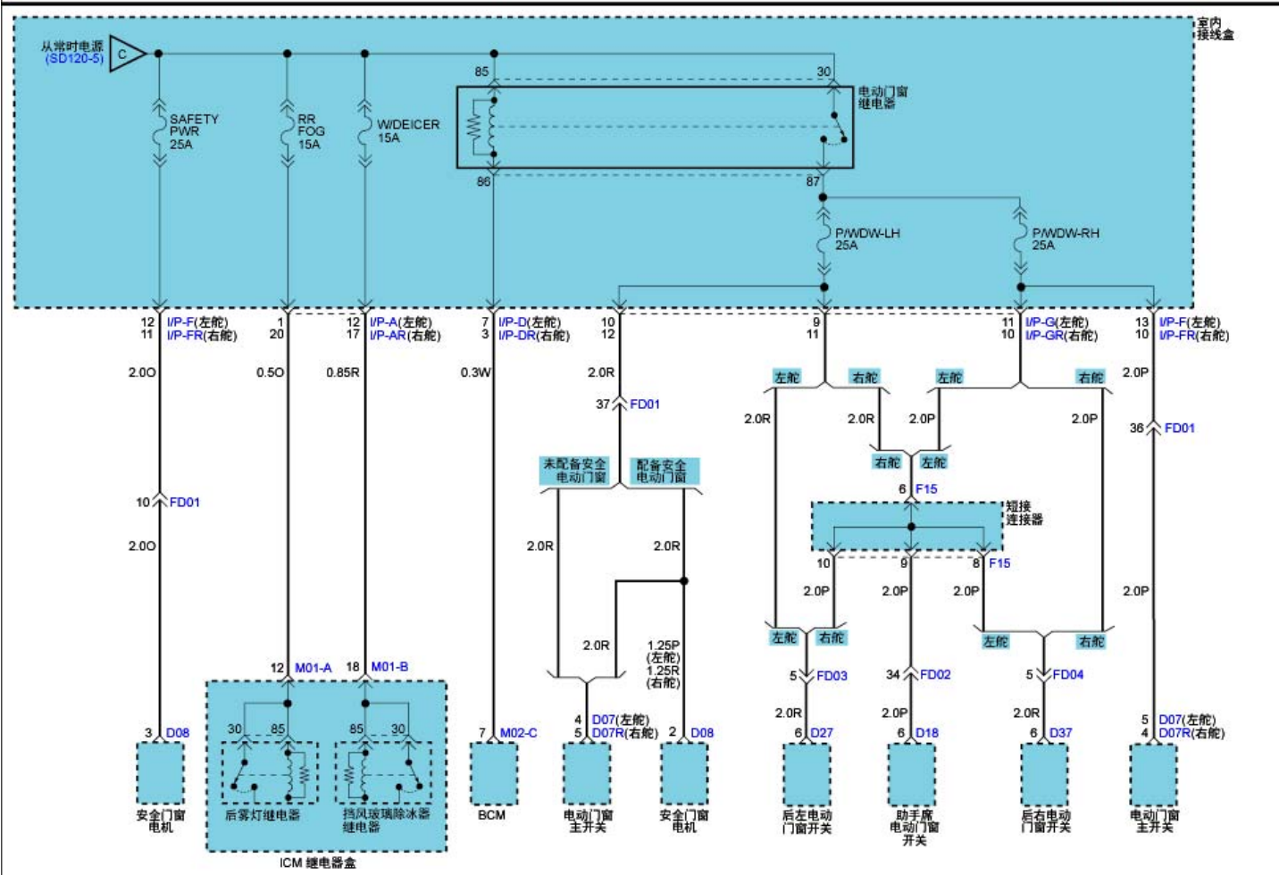
室内保险丝分布 (6)
